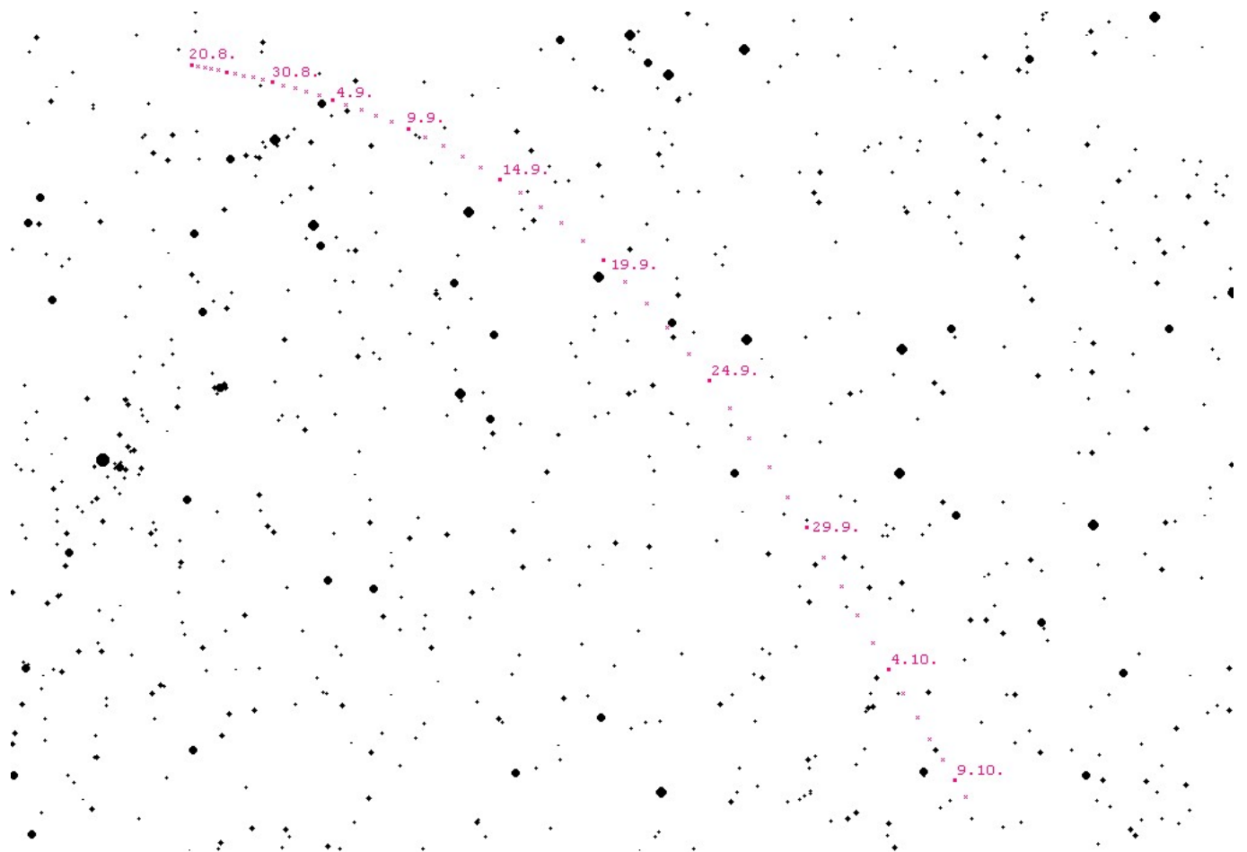
Bewegung des Kometen C/2018 W2 (Africano) vom 20.8.19 bis 10.10.19
